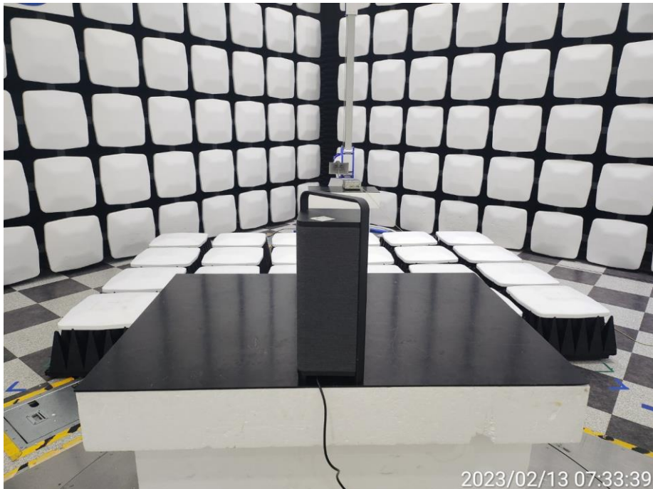
[CHARGE 모드_후면]
