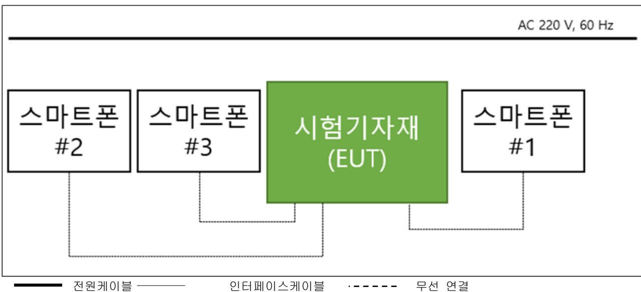
[BT + Wi-Fi 2.4 GHz 모드_EMI/EMS]
