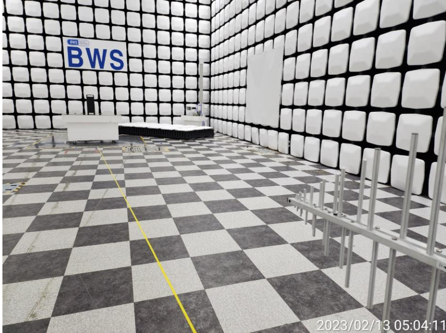
[BT + Wi-Fi 2.4 GHz 모드_전면]
