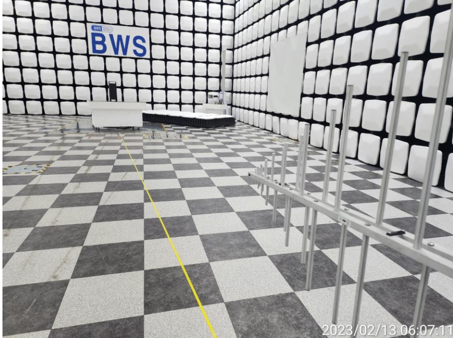
[CHARGE 모드_전면]
